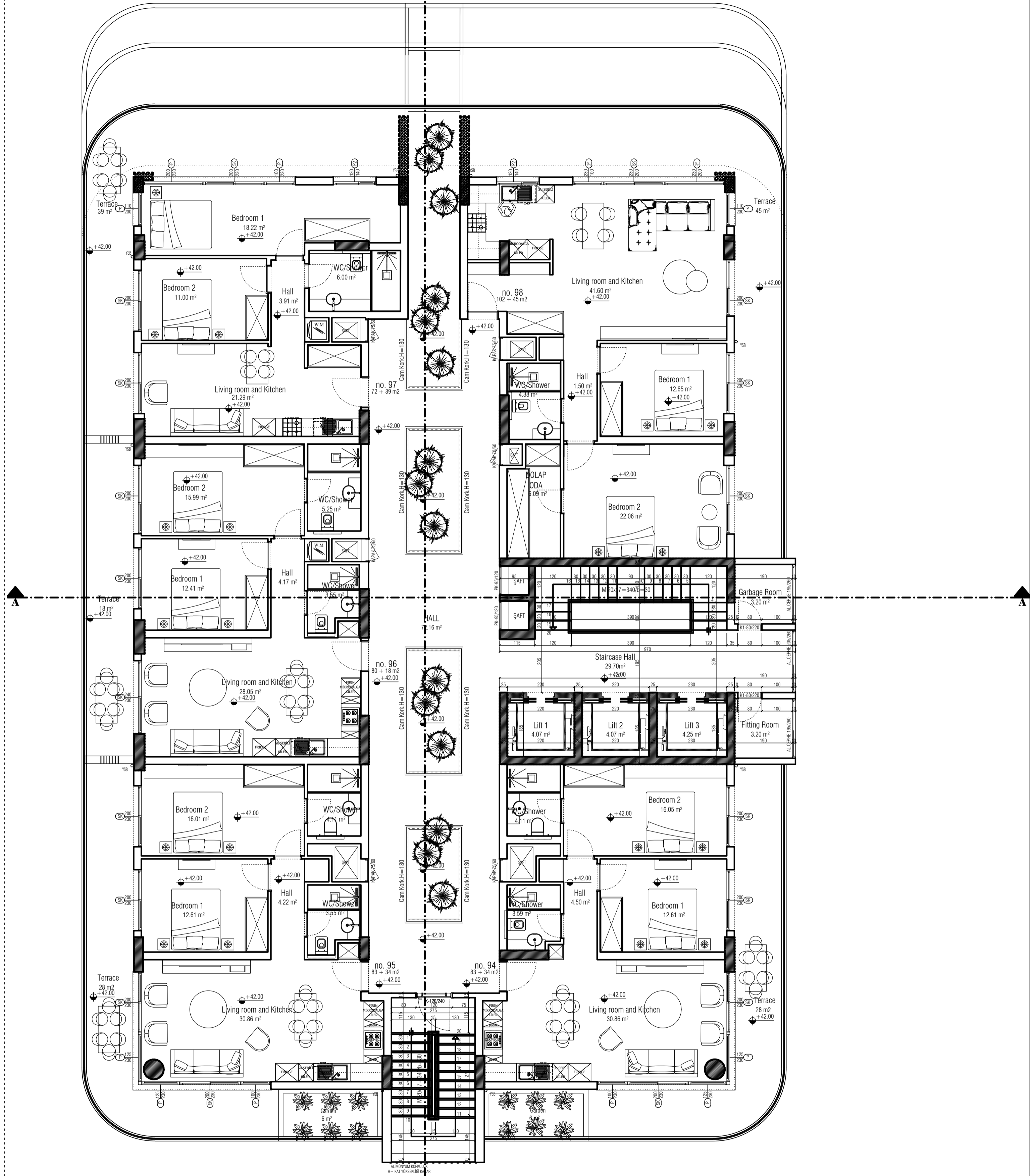
12th FLOOR (+42.00 KODU) 12. KAT PLANI ÖLÇEK 1/100
