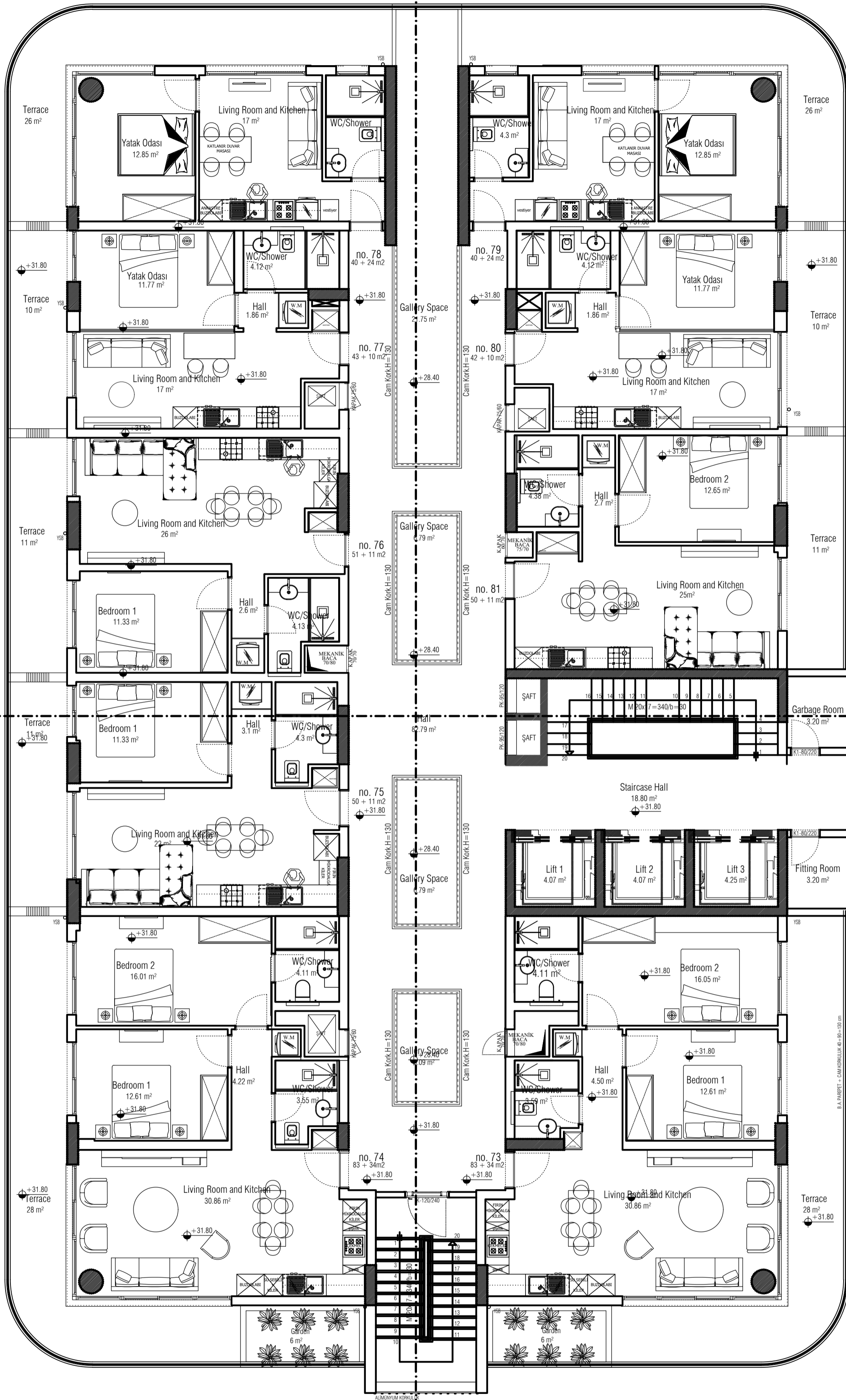
9th FLOOR (+31.80 KODU) 9. KAT PLANI ÖLÇEK 1/100
