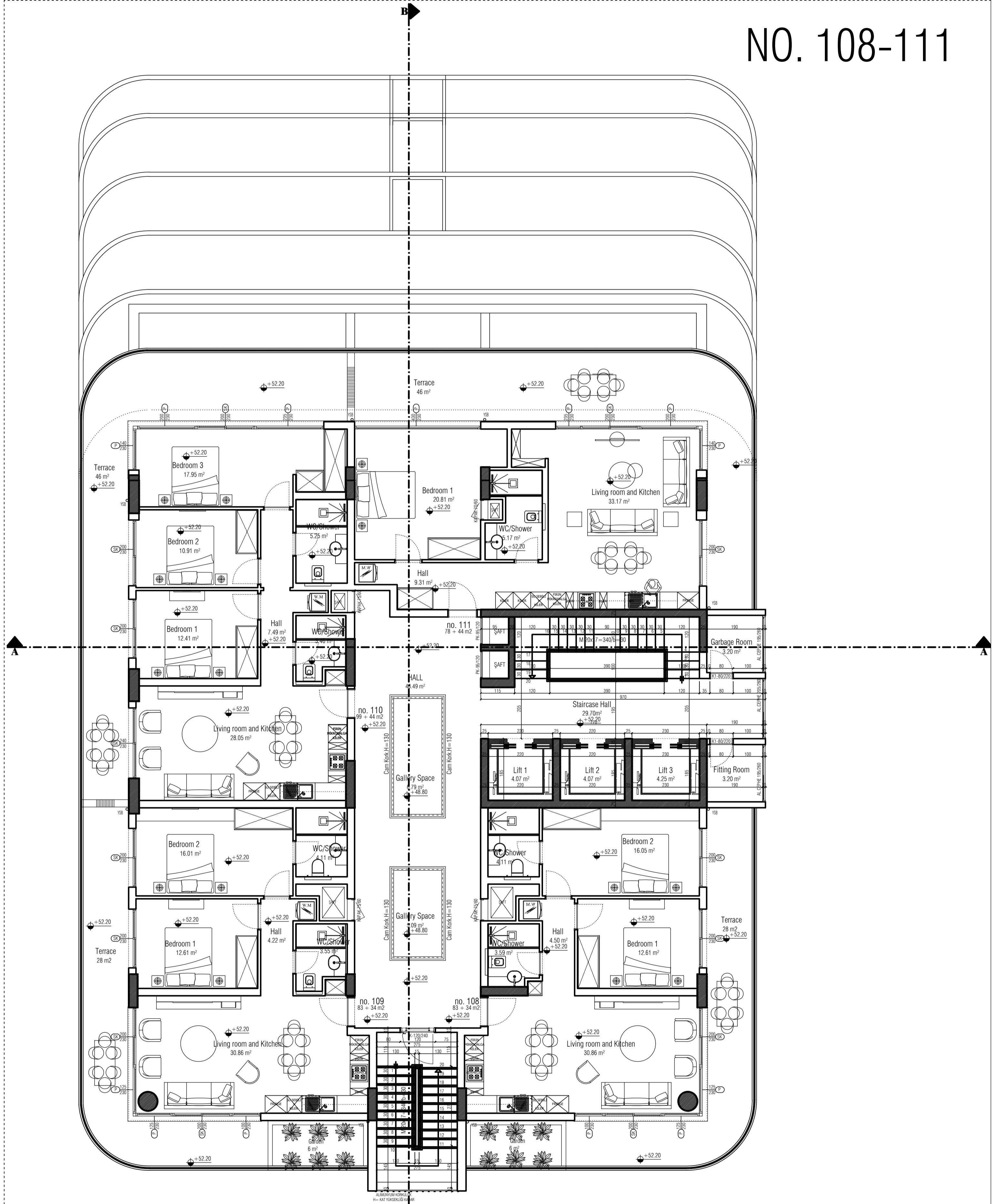
15th FLOOR (+52.20 KODU) 15. KAT PLANI ÖLÇEK 1/100
