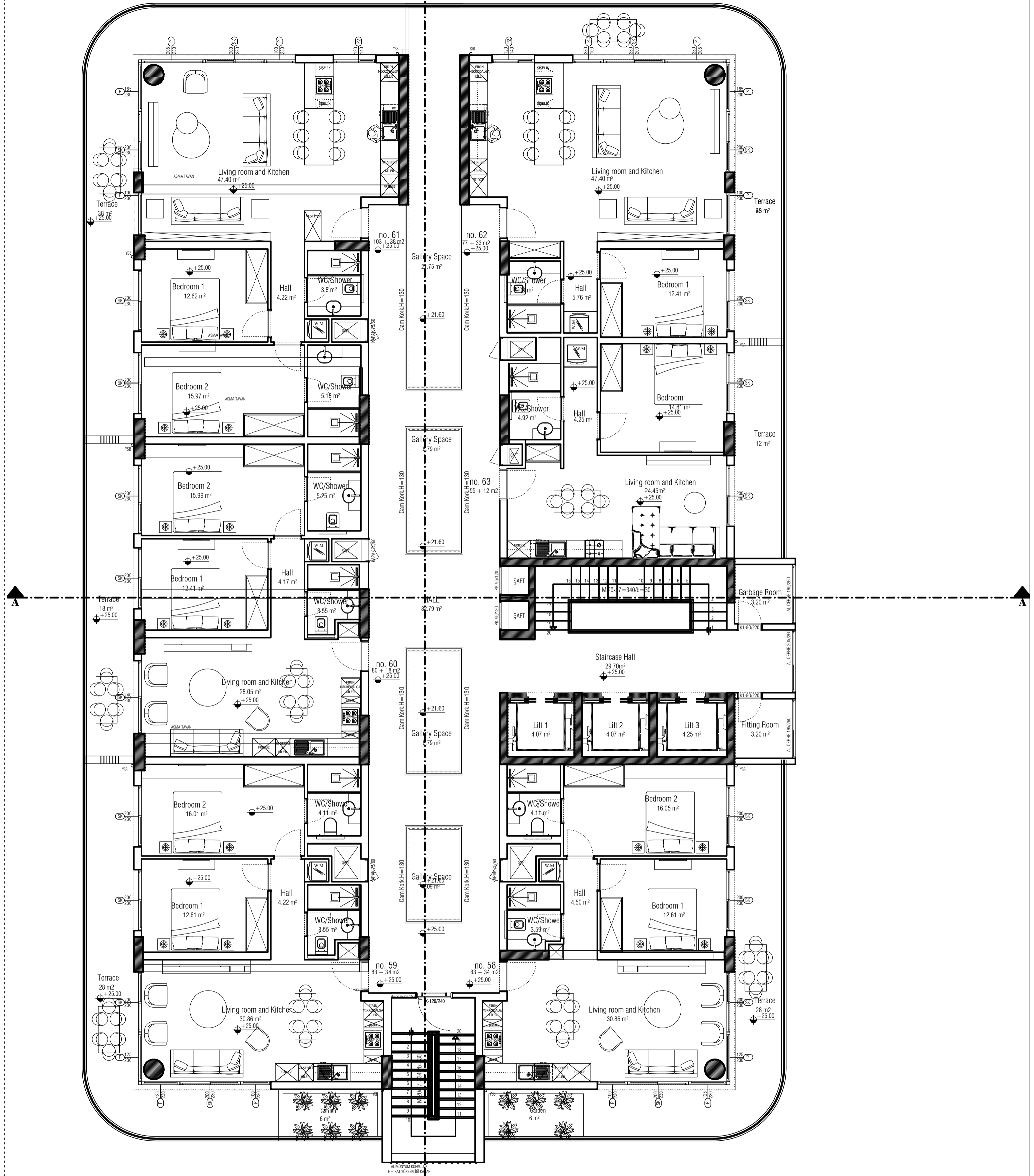
7th FLOOR (+25.00 KODU) 7. KAT PLANI ÖLÇEK 1/100
