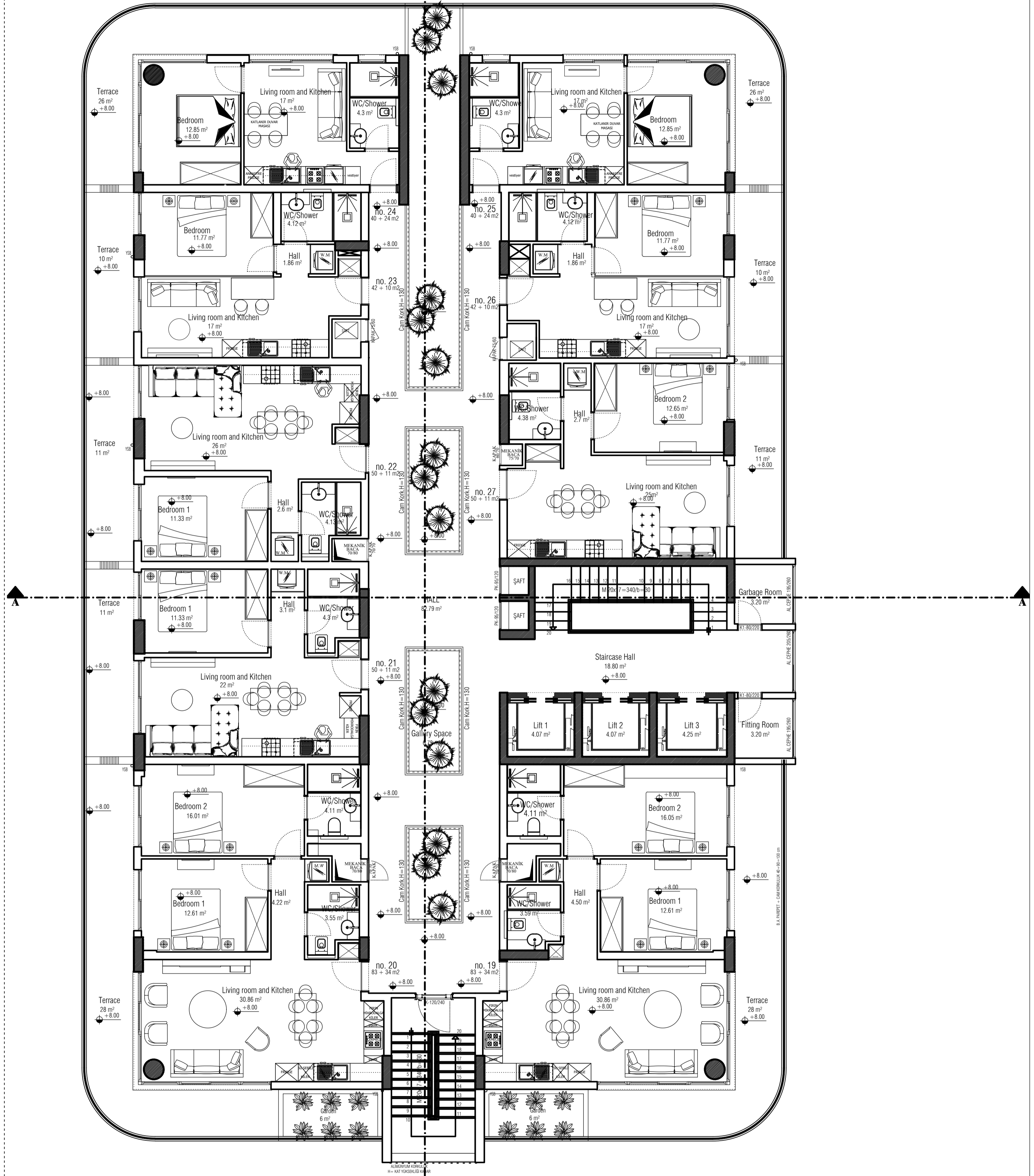
2nd FLOOR (+8.00 KODU) 2. KAT PLANI ÖLÇEK 1/100
