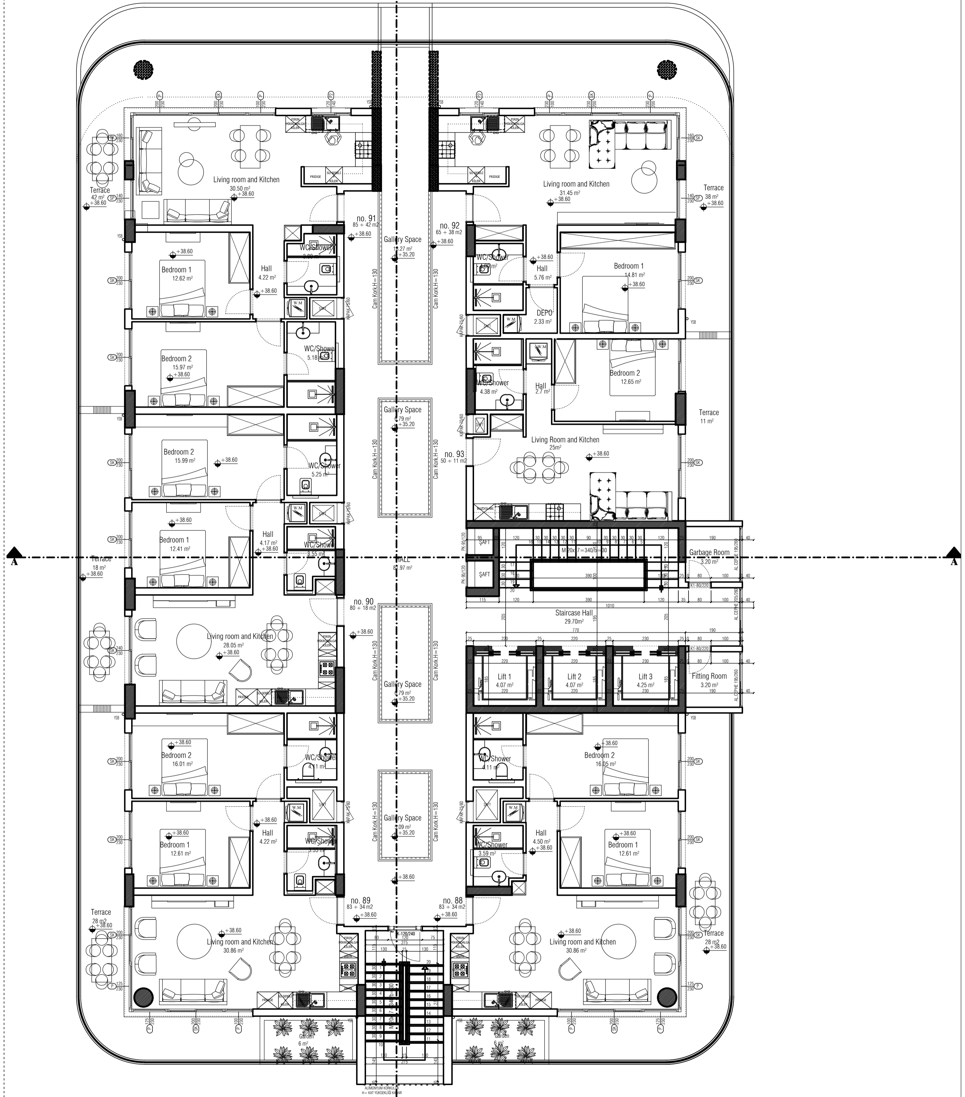
11th FLOOR (+38.60 KODU) 11. KAT PLANI ÖLÇEK 1/100
