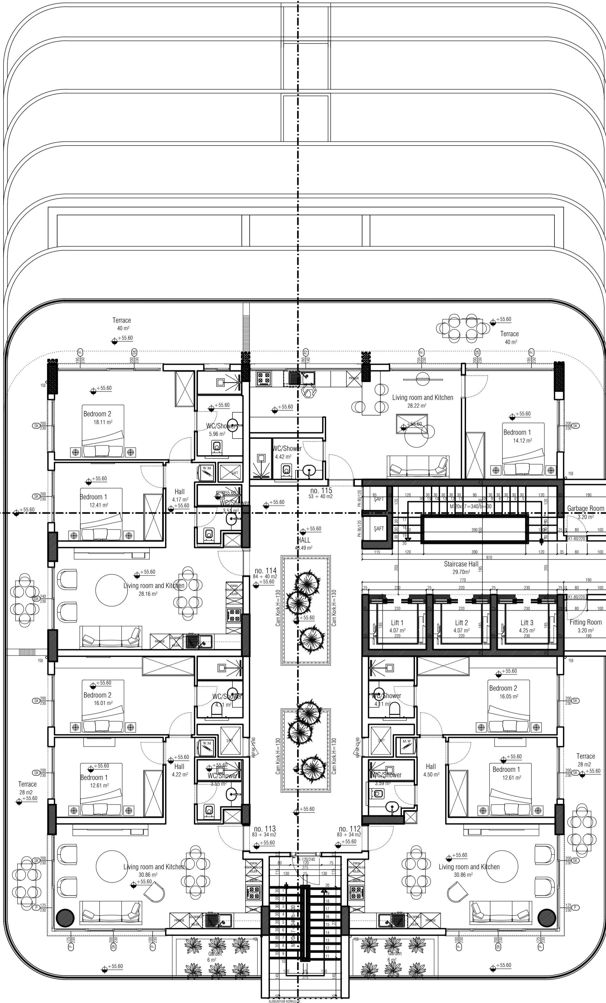
16th FLOOR (+55.60 KODU) 16. KAT PLANI ÖLÇEK 1/100
