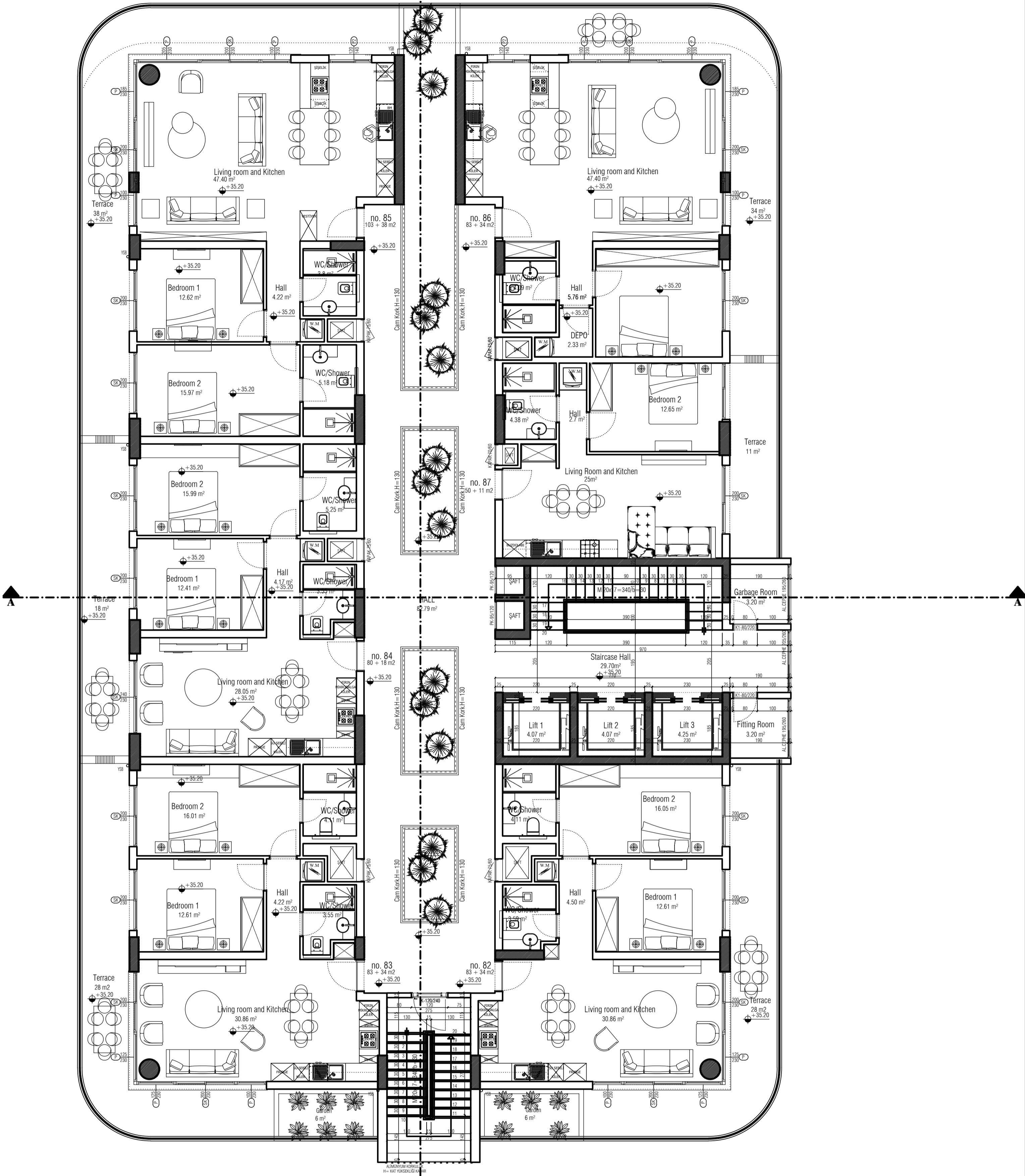
10th FLOOR (+35.20 KODU) 10. KAT PLANI ÖLÇEK 1/100
