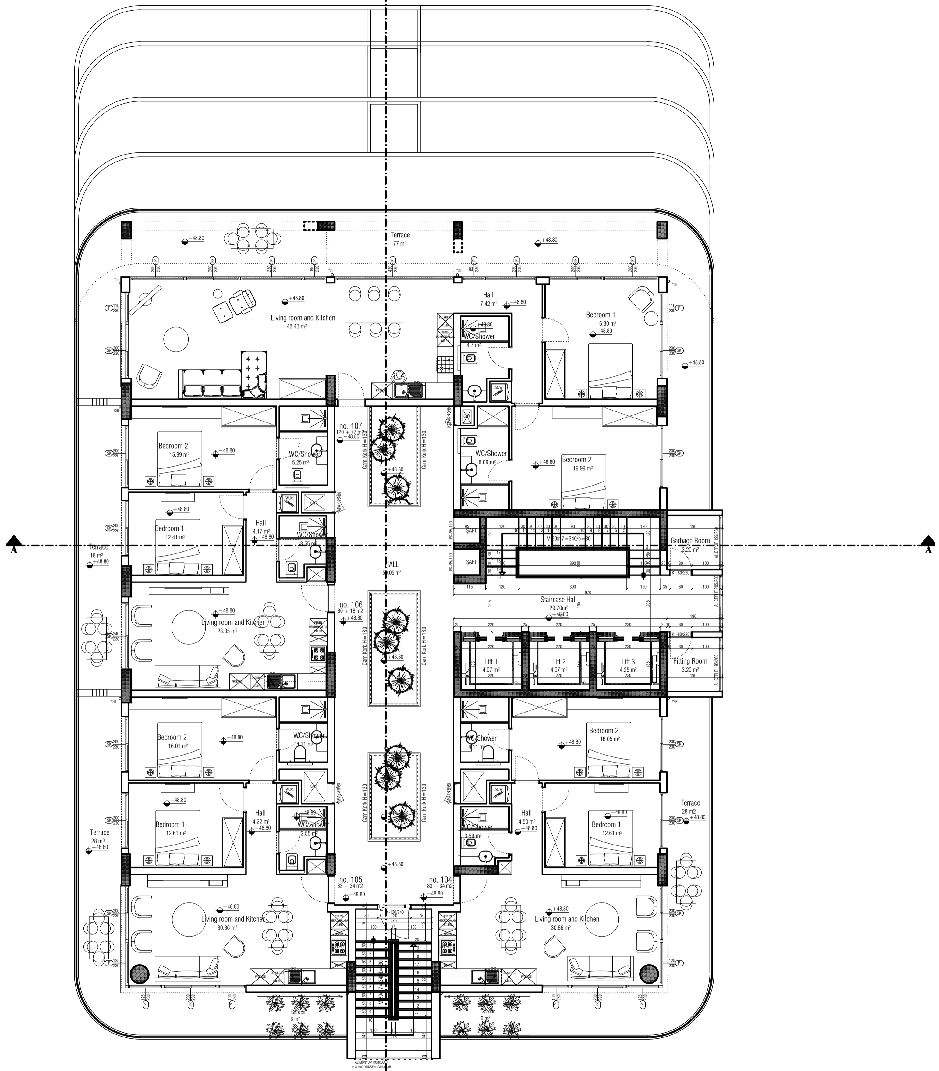
14th FLOOR (+48.80 KODU) 14. KAT PLANI ÖLÇEK 1/100
