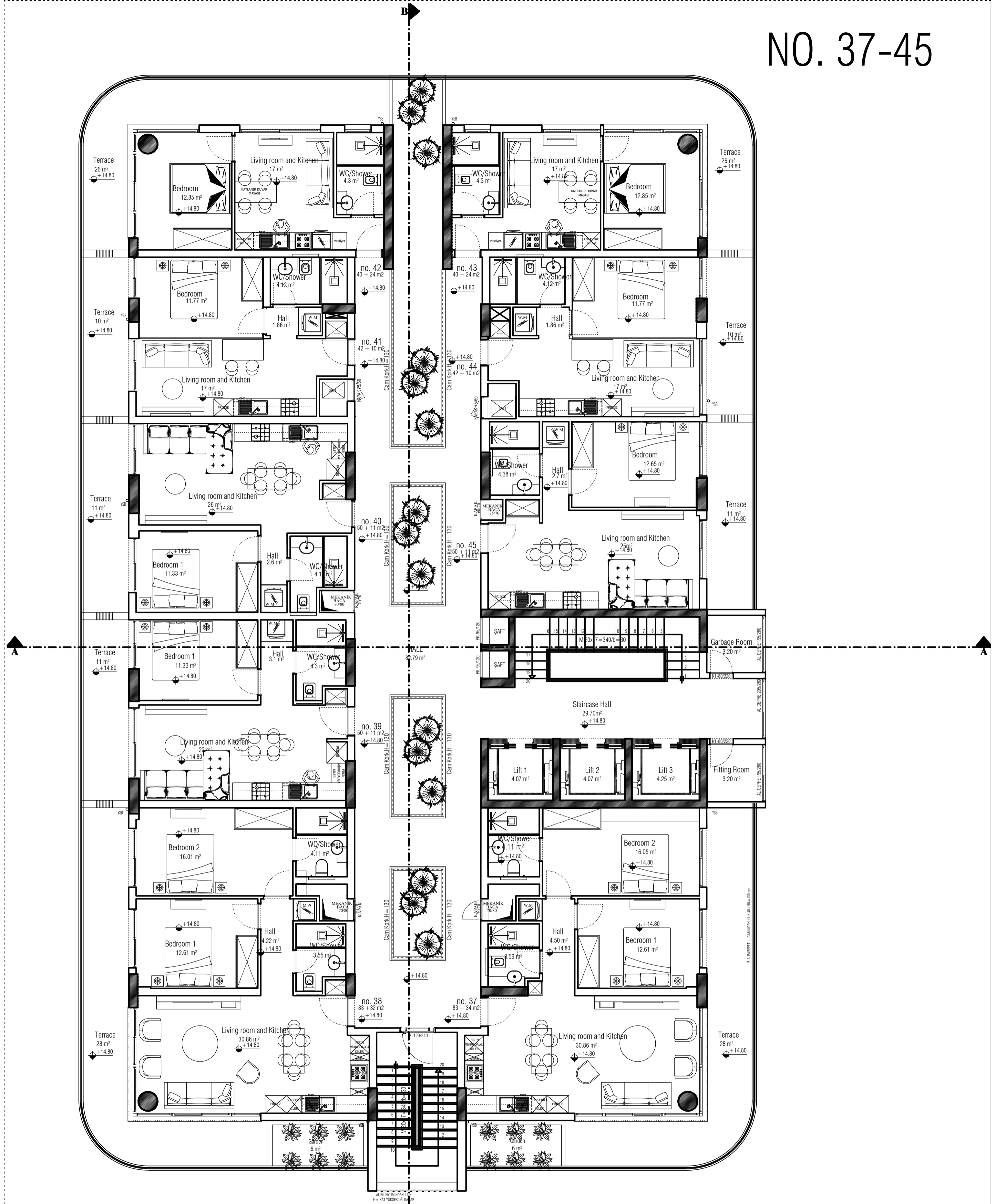
4th FLOOR (+14.80 KODU) 4. KAT PLANI ÖLÇEK 1/100
