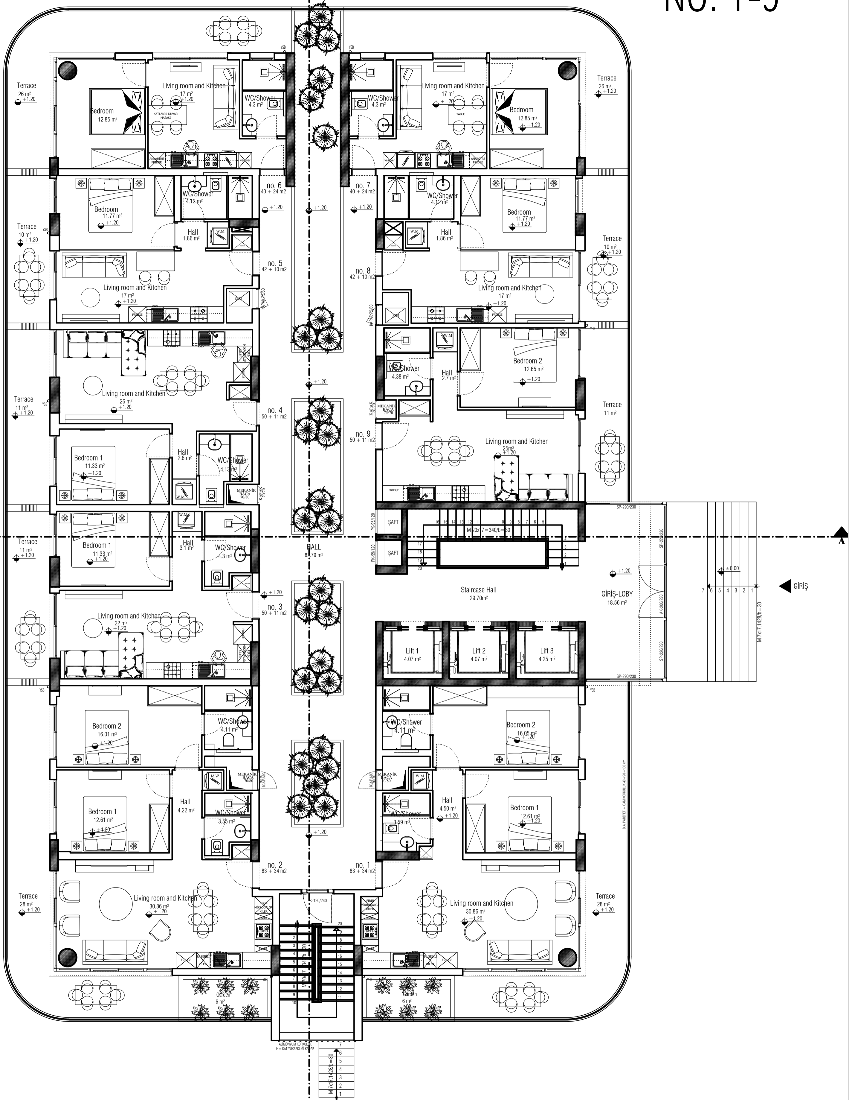
(+1.20 KODU) ZEMİN KAT PLANI ÖLÇEK 1/100 GROUND FLOOR
