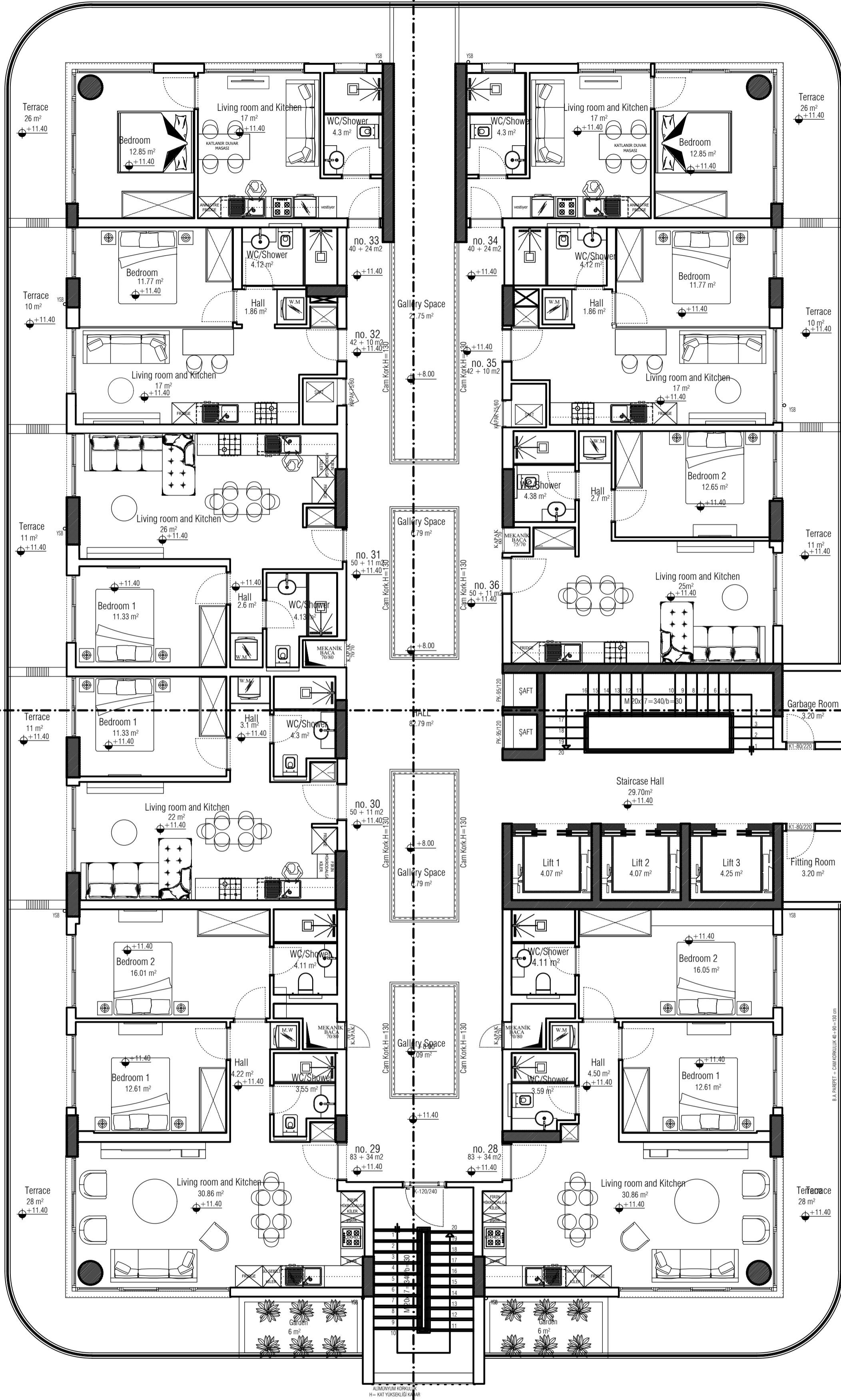
3rd FLOOR (+11.40 KODU) 3. KAT PLANI ÖLÇEK 1/100
