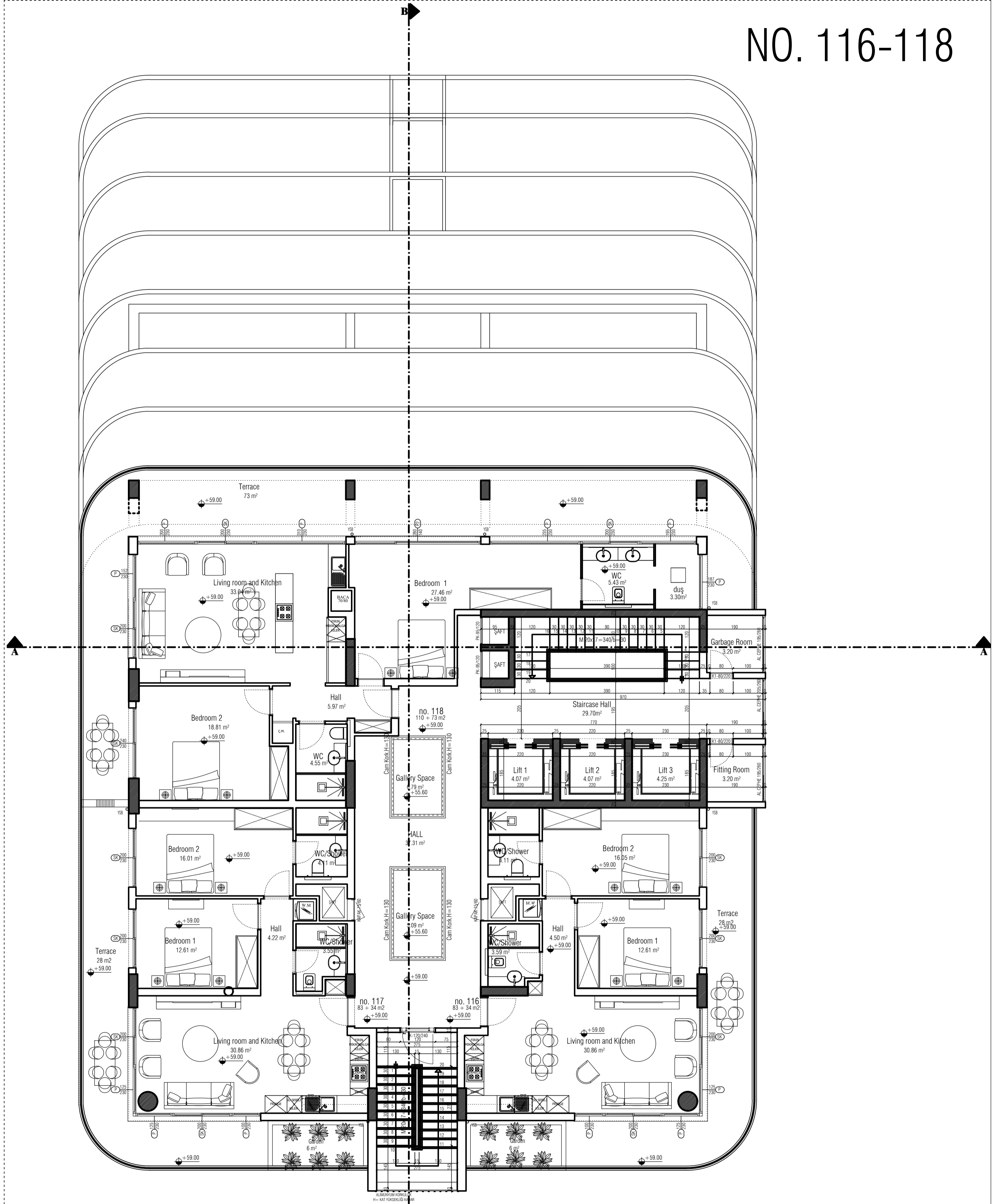
17th FLOOR (+59.00 KODU) 17. KAT PLANI ÖLÇEK 1/100
