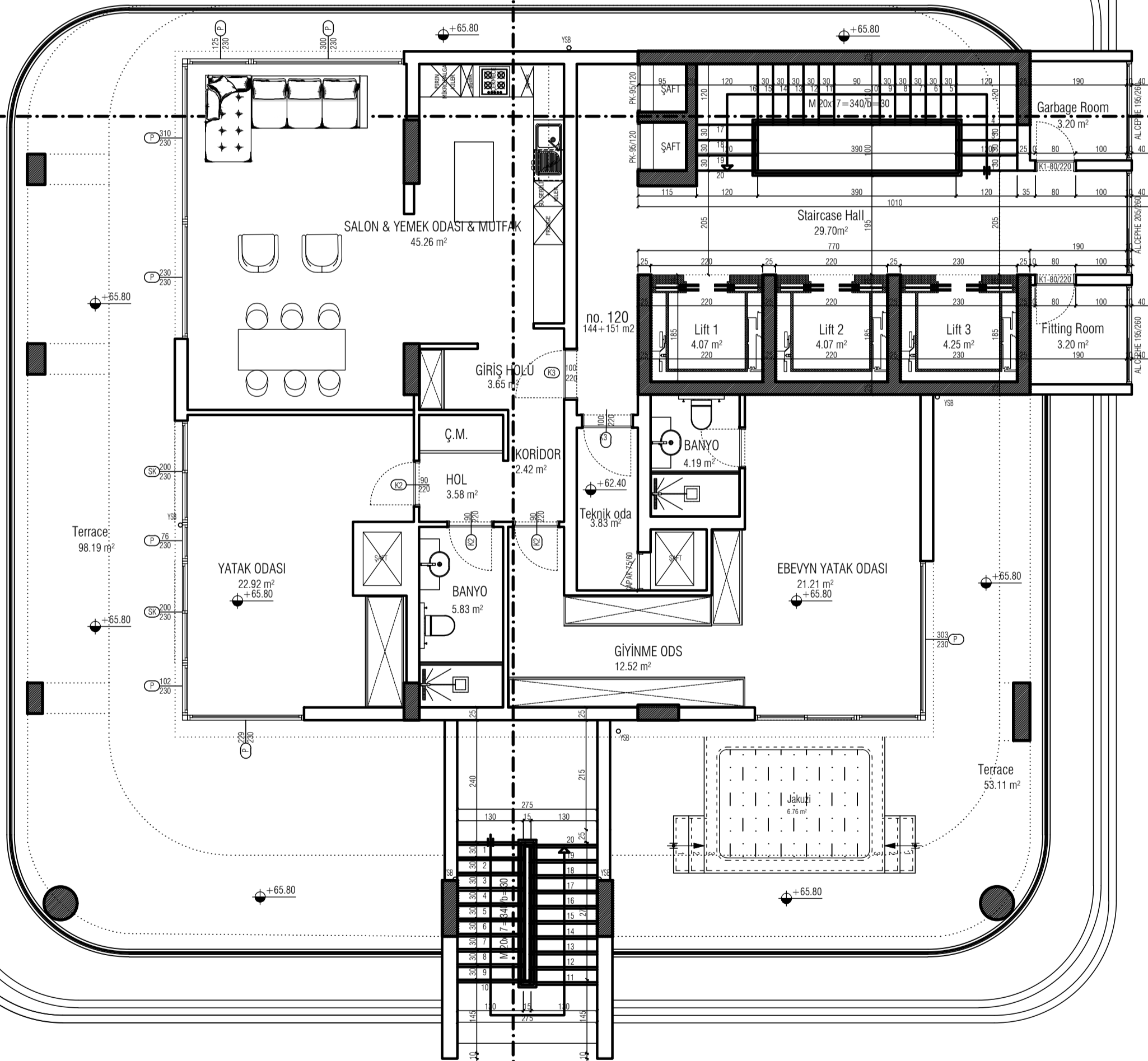
19th FLOOR (+65.80 KODU) 19. KAT PLANI ÖLÇEK 1/100
